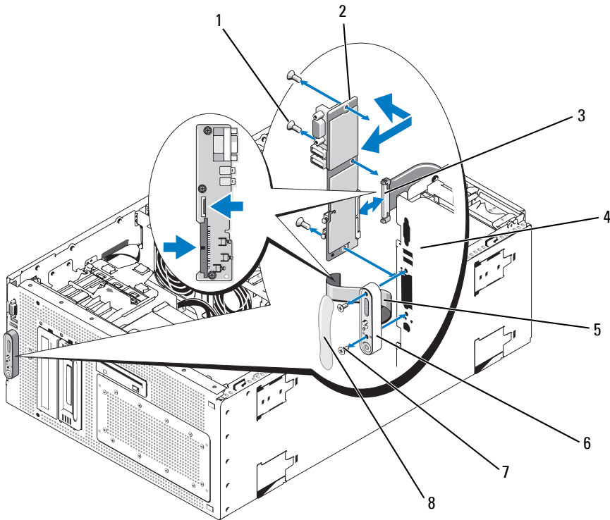
그림 3-27. 제어판 조립품 분리
