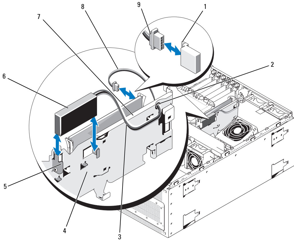
그림 3-25. SAS RAID 컨트롤러 보조 카드 전지 장착
