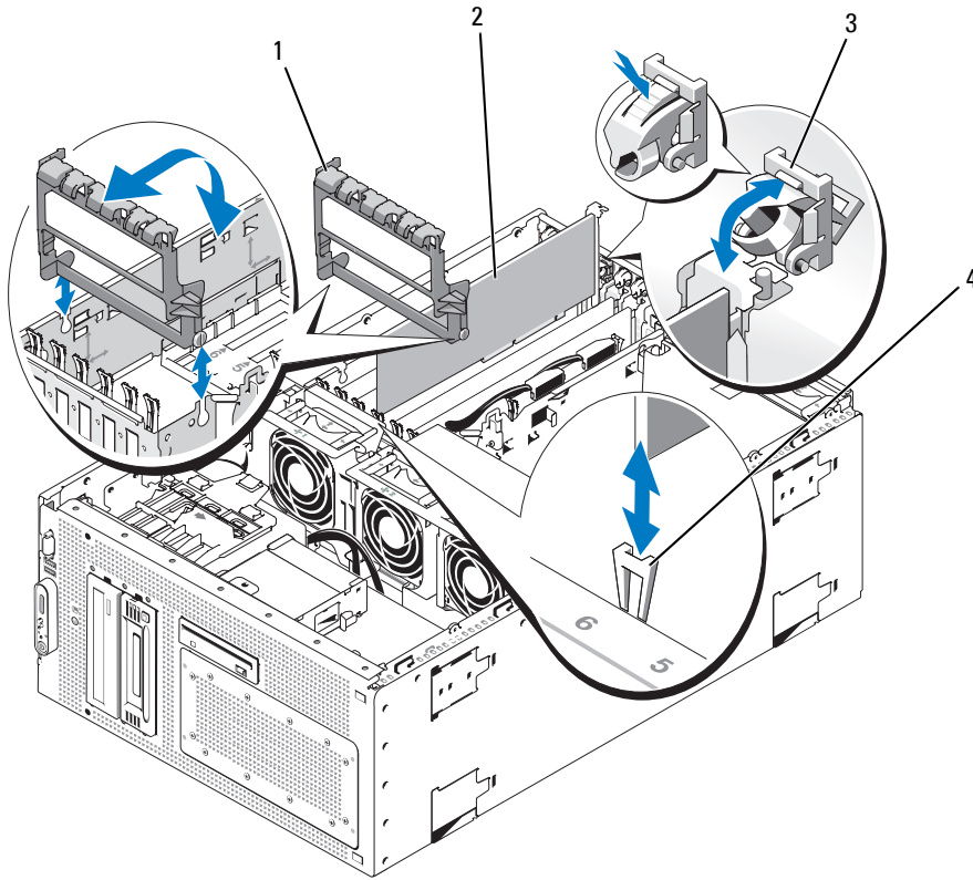
그림 3-9. 확장 카드 설치 및 분리
