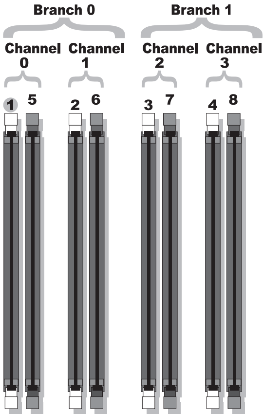
그림 3-20. DIMM 소켓
