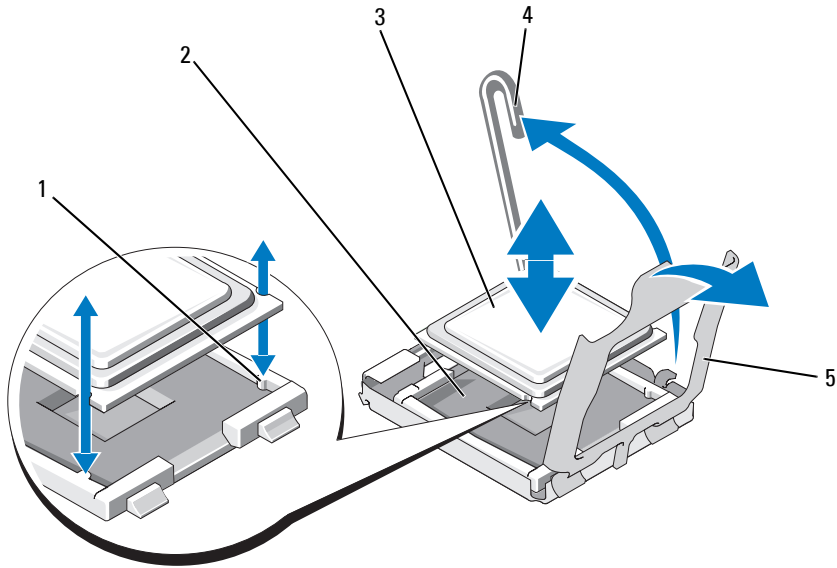
그림 3-24. 프로세서 설치 및 분리
