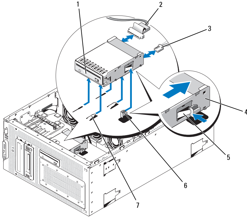
그림 3-16. 디스켓 드라이브 설치 및 분리
