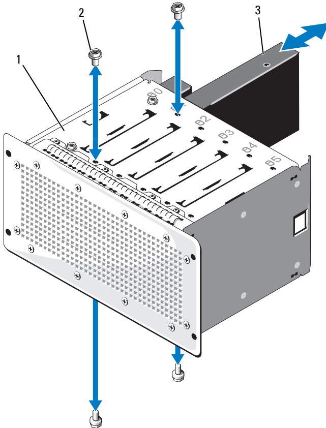
그림 3-11. 하드 드라이브 분리 및 설치
