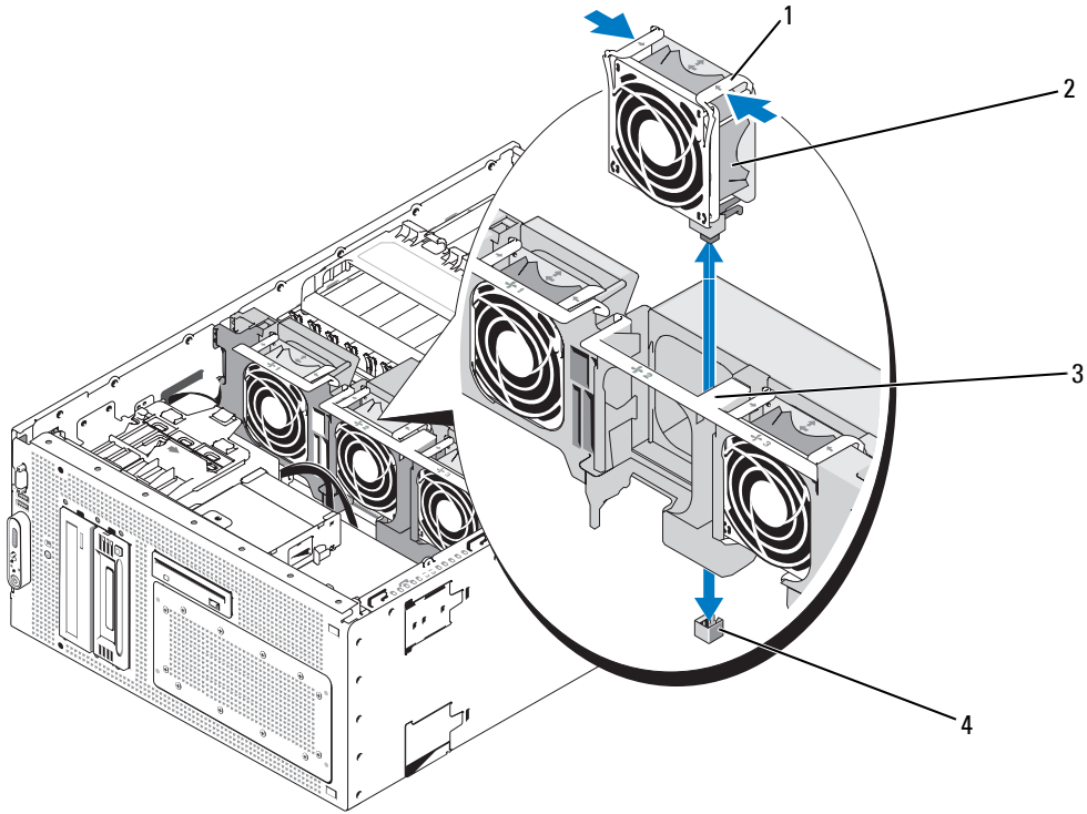
그림 3-6. 팬 브래킷에서 팬 설치 및 분리
