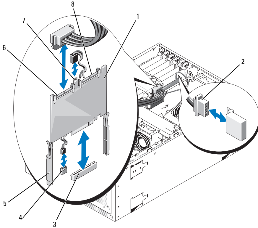
그림 3-26. SAS RAID 컨트롤러 보조 카드 설치 및 분리
