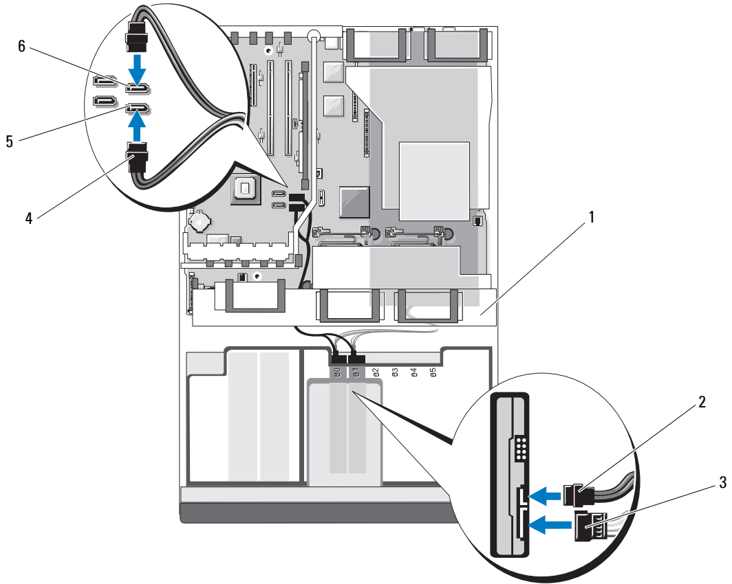
그림 3-12. 2 개의 하드 드라이브 구성 (시스템 보드의 내장형 SATA)
