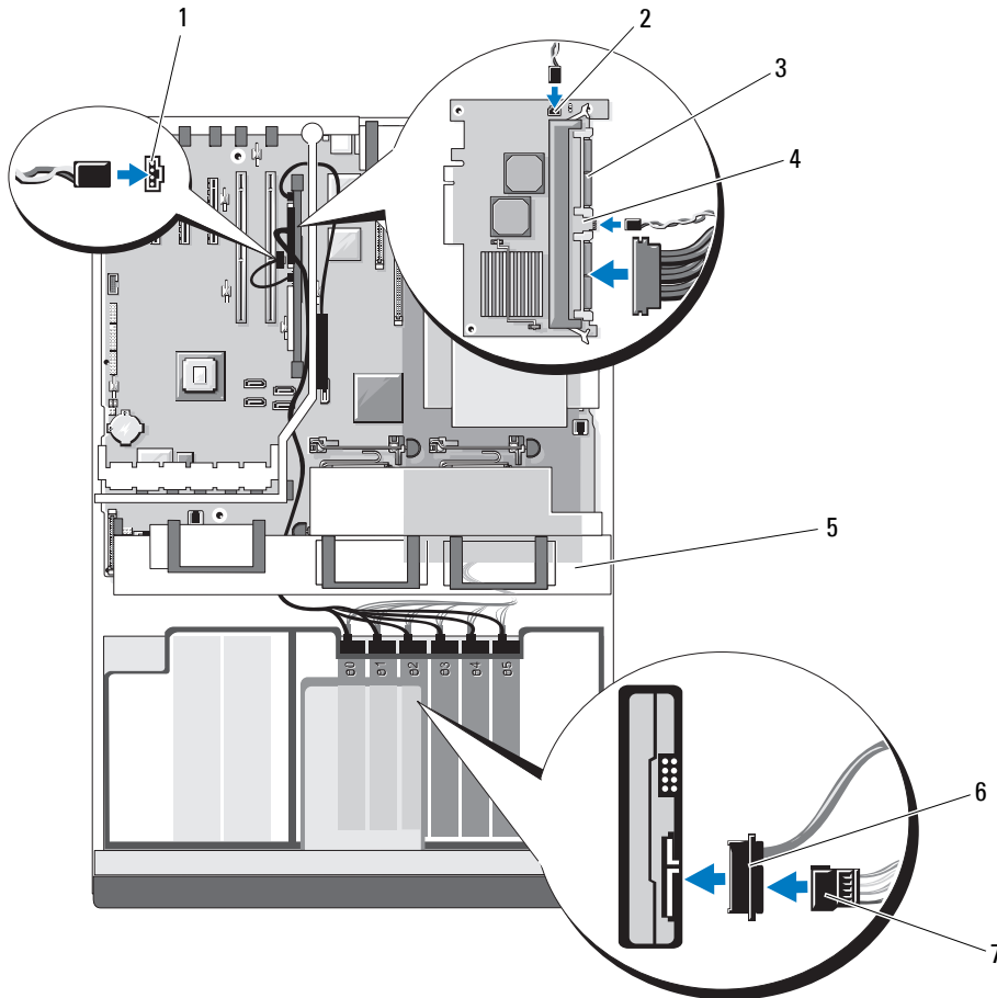
그림 3-14. 6 하드 드라이브 구성 (SAS 컨트롤러 보조 카드)
