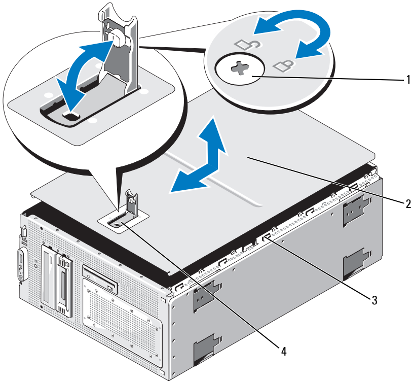
그림 3-3. 시스템 덮개 설치 및 분리
