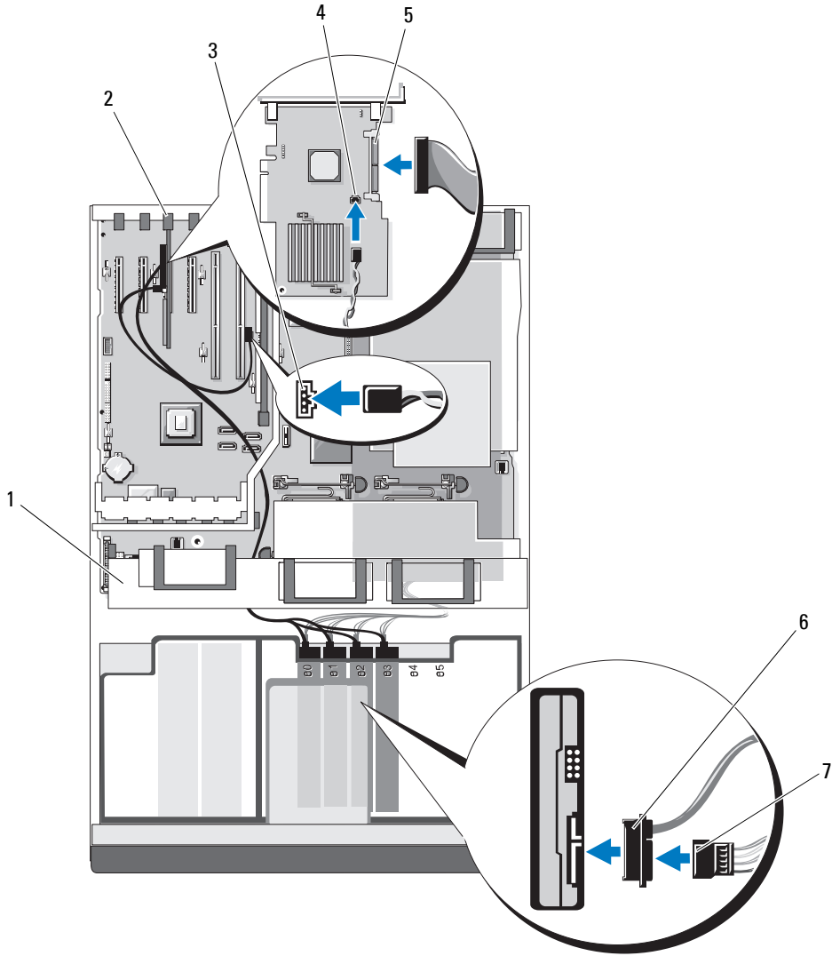
그림 3-13. 4 하드 드라이브 구성 (SAS 컨트롤러 카드)
