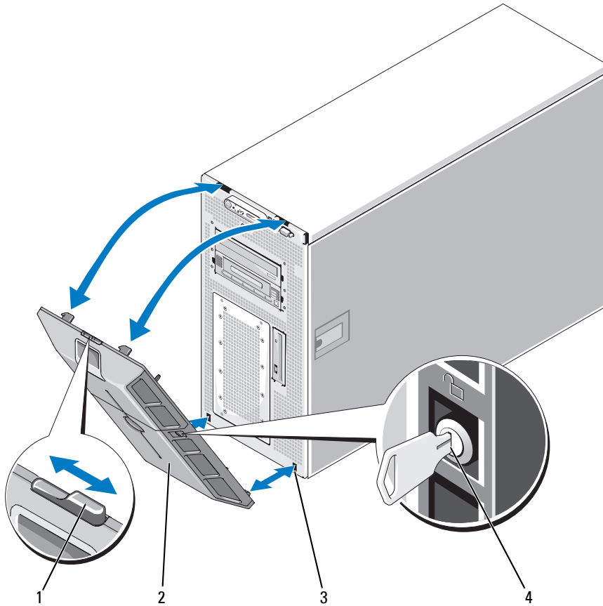
그림 3-2. 베젤 설치 및 분리
