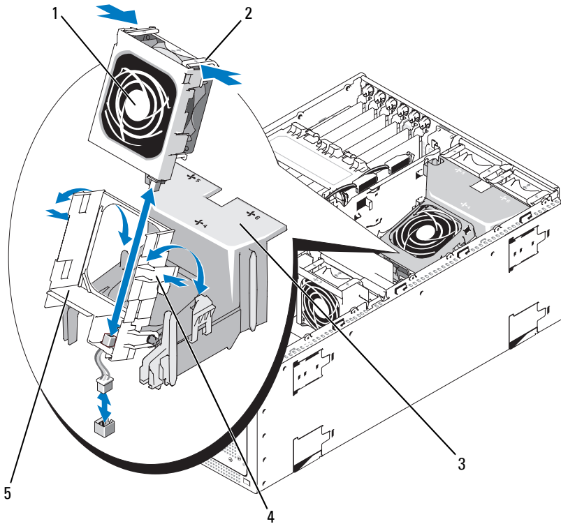
그림 3-7. 냉각 덮개 팬 분리 및 장착
