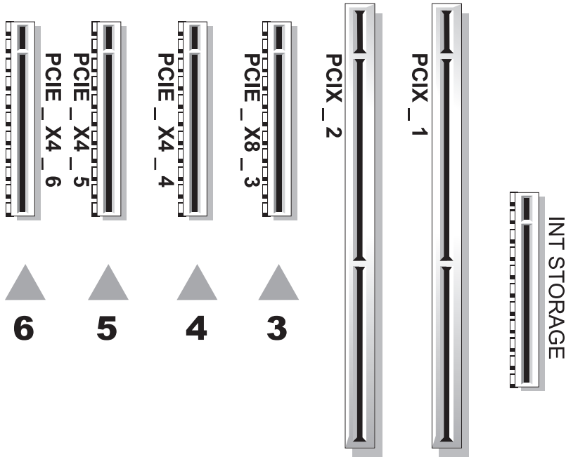
그림 3-8. 확장 슬롯
