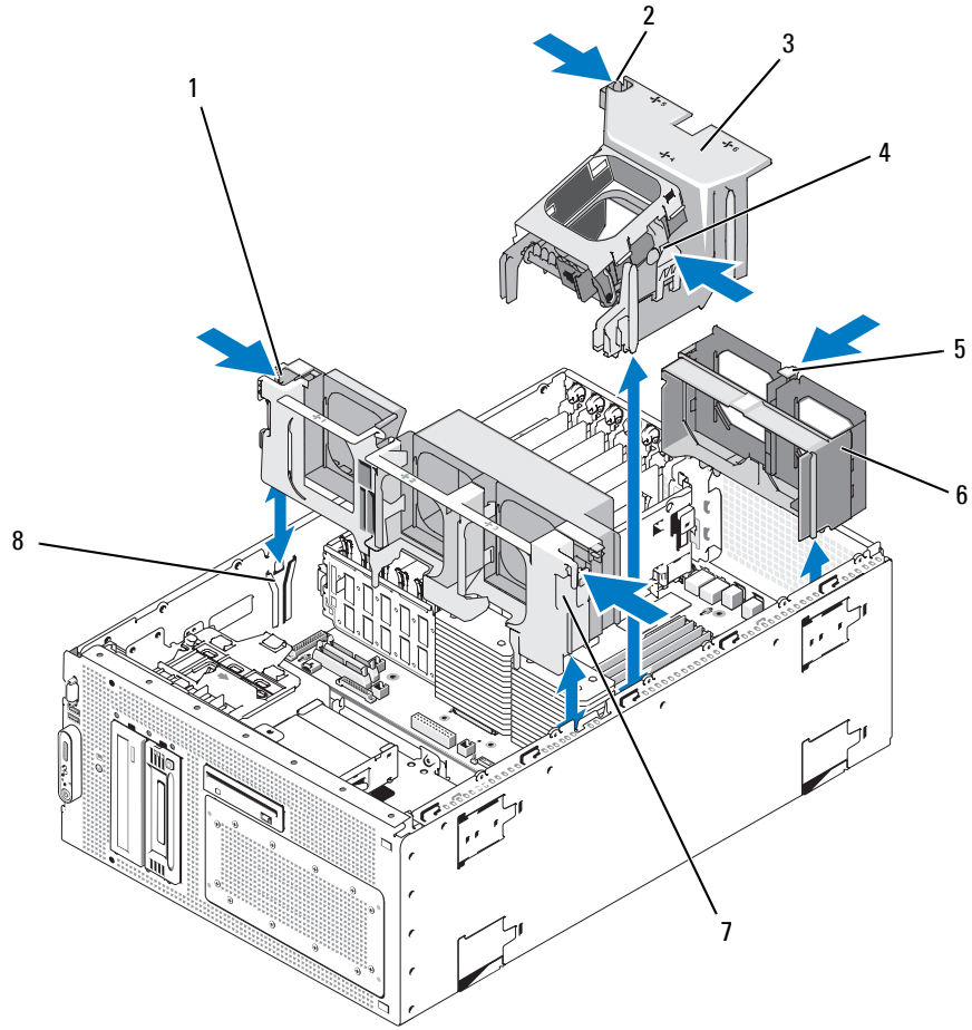
그림 3-19. 팬 브래킷 및 냉각 덮개 설치 및 분리
