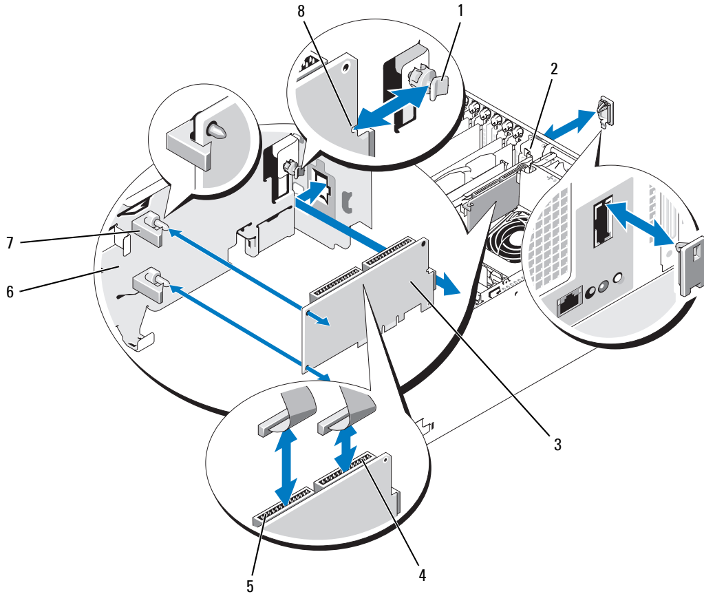
그림 3-22. RAC 카드 설치
