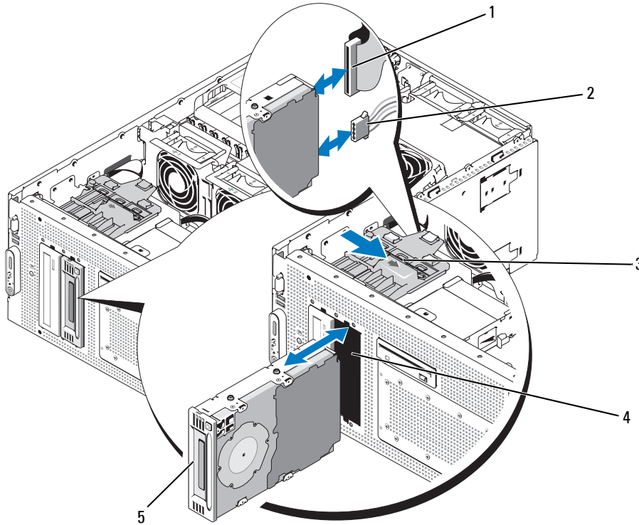
그림 3-15. Half-Height 테이프 백업 단원 또는 광학 드라이브 설치 및 분리
