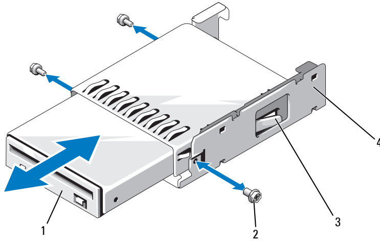
그림 3-17. 드라이브 캐리어에 디스켓 드라이브 설치
