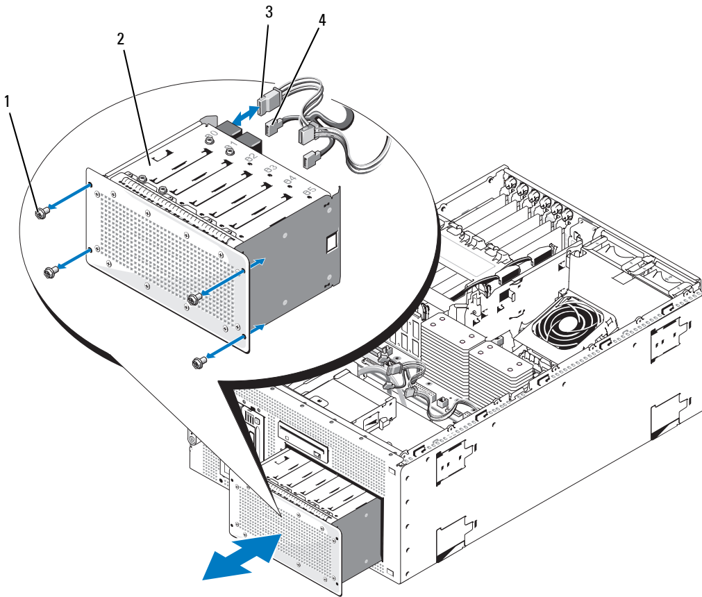
그림 3-10. 하드 드라이브 베이 분리 및 설치
