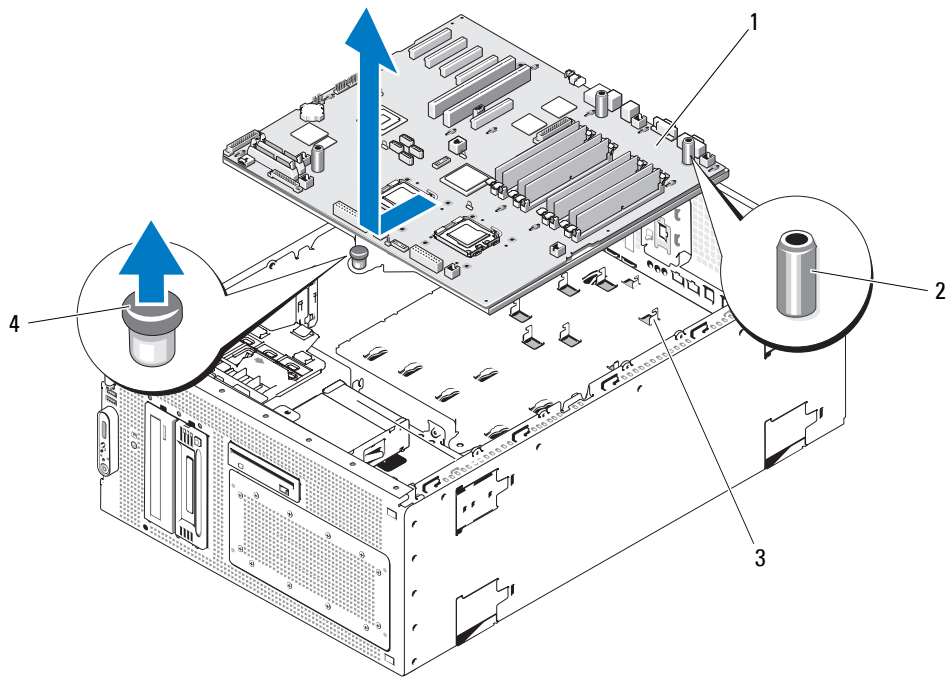
그림 3-28. 시스템 보드 분리
