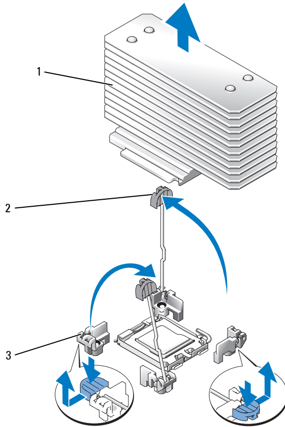
1 방열판 2 방열판 고정 레버 (2개) 3 고정 레버 래치
