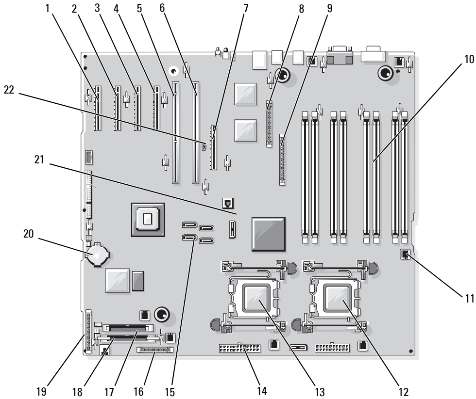
그림 6-2. 시스템 보드 커넥터
