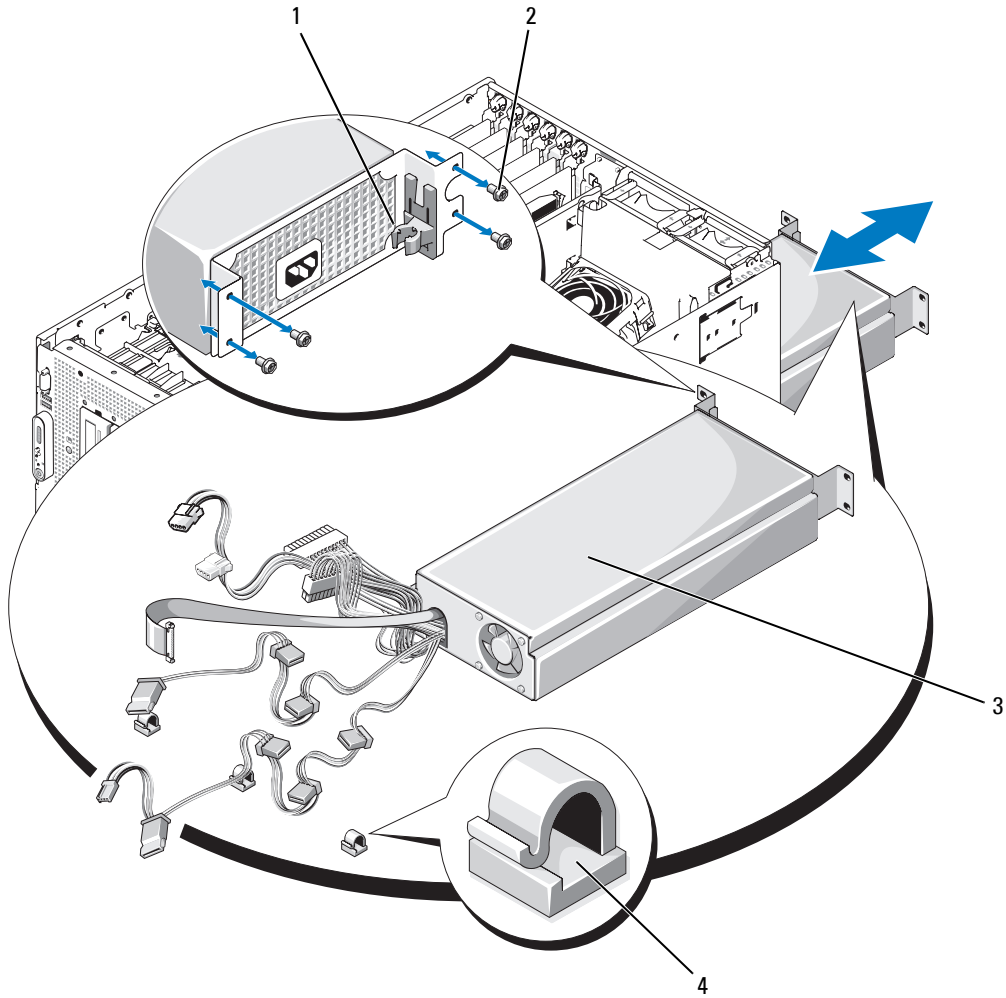
그림 3-4. 전원 공급 장치 설치 및 분리
